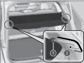
1 Ράβδος στερέωσης
